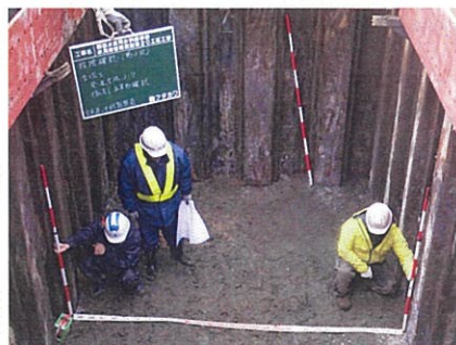
発進立坑出来形確認
