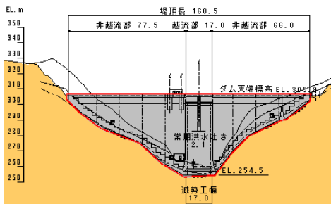
ダムの正面図(下流側)
