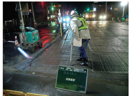
路面切削高確認 県管理道路舗装補修工 工事 発注者:富山県富山土木センター 〔設計積算・施工管理〕
